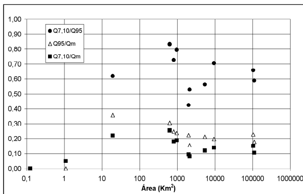
Figura 22. Índices regionais para a região do rio Ijuí.
