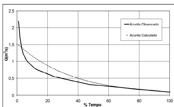
Figura 18. Curva de permanência regionalizada para a bacia Azurita – 21,7 km 2 (Paraopeba).
