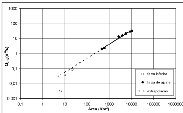
Figura 21. Regionalização da Q_{7,10} (bacia do rio Paraopeba).
