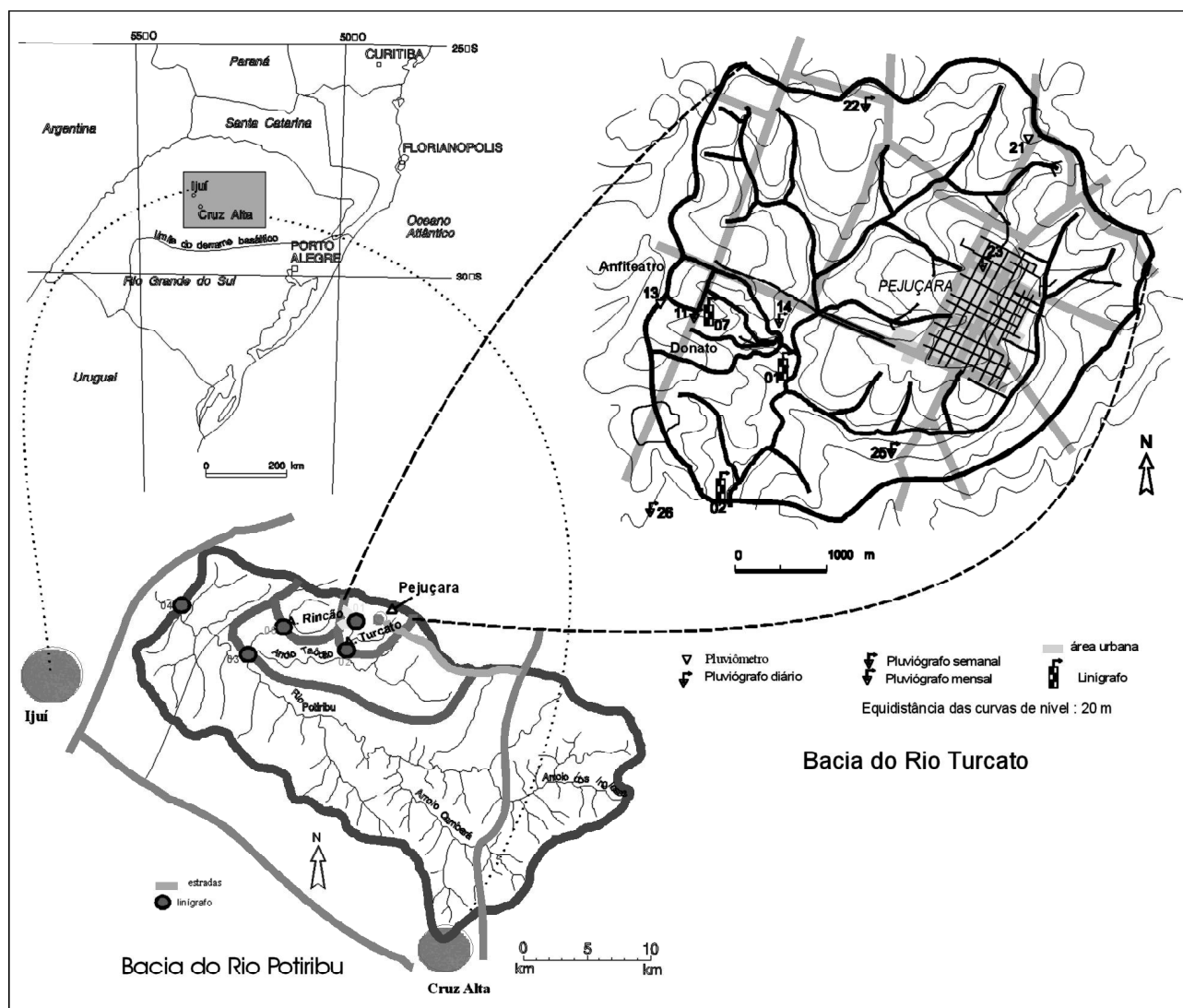
Figura 2. Bacia do rio Potiribu, englobando as bacias do Turcato, Donato e Anfiteatro (Castro et al., 2000).
