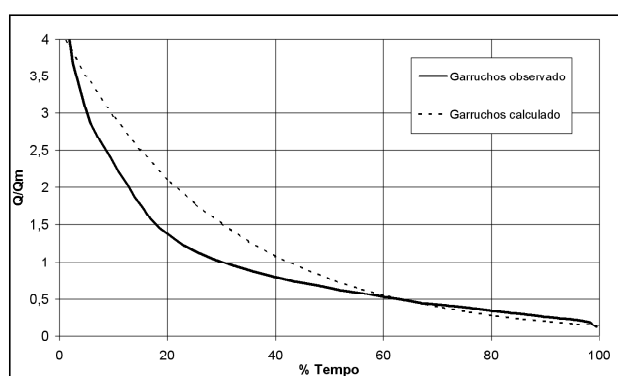
Figura 16. Curva de permanência regionalizada para Garruchos (104.162 km 2 ), no rio Uruguai.
