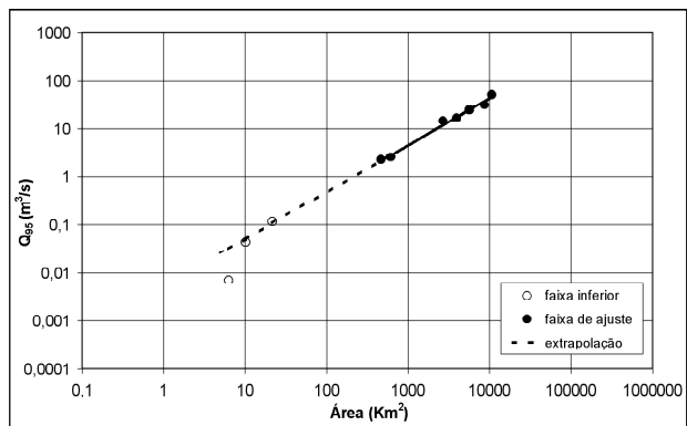
Figura 14. Regionalização do Q 95 (Paraopeba).
