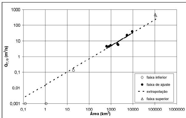
Figura 20. Regionalização da Q_{7,10} (região do rio Ijuí).
