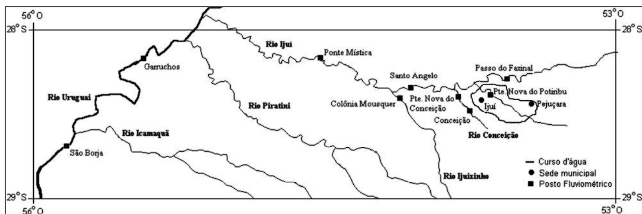
Figura 1. Localização dos postos fluviométricos da região do Ijuí (Modificado de BRASIL, 2000).
