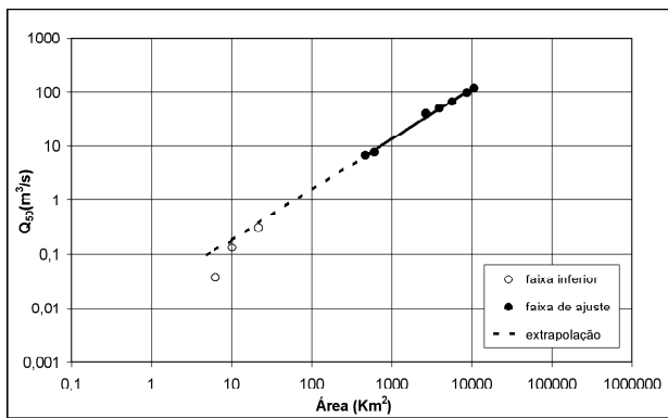
Figura 12. Regionalização do Q 50 (Paraopeba).
