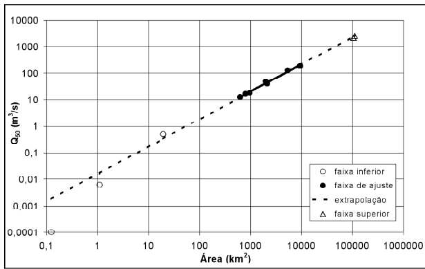
Figura 11. Regionalização do Q 50 (Ijuí).
