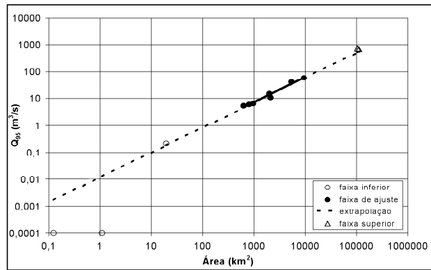
Figura 13. Regionalização do Q 95 (Ijuí).
