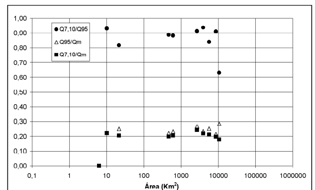
Figura 23. Índices regionais para a bacia do rio Paraopeba.
