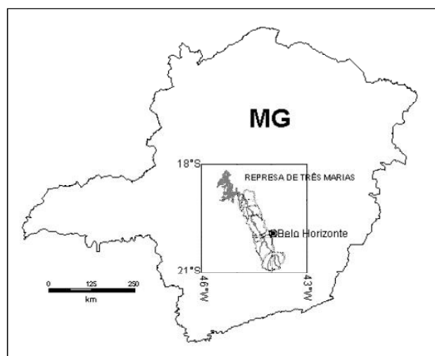
Figura 3. Localização da bacia do rio Paraopeba em Minas Gerais (Schvartzman, 2000).
