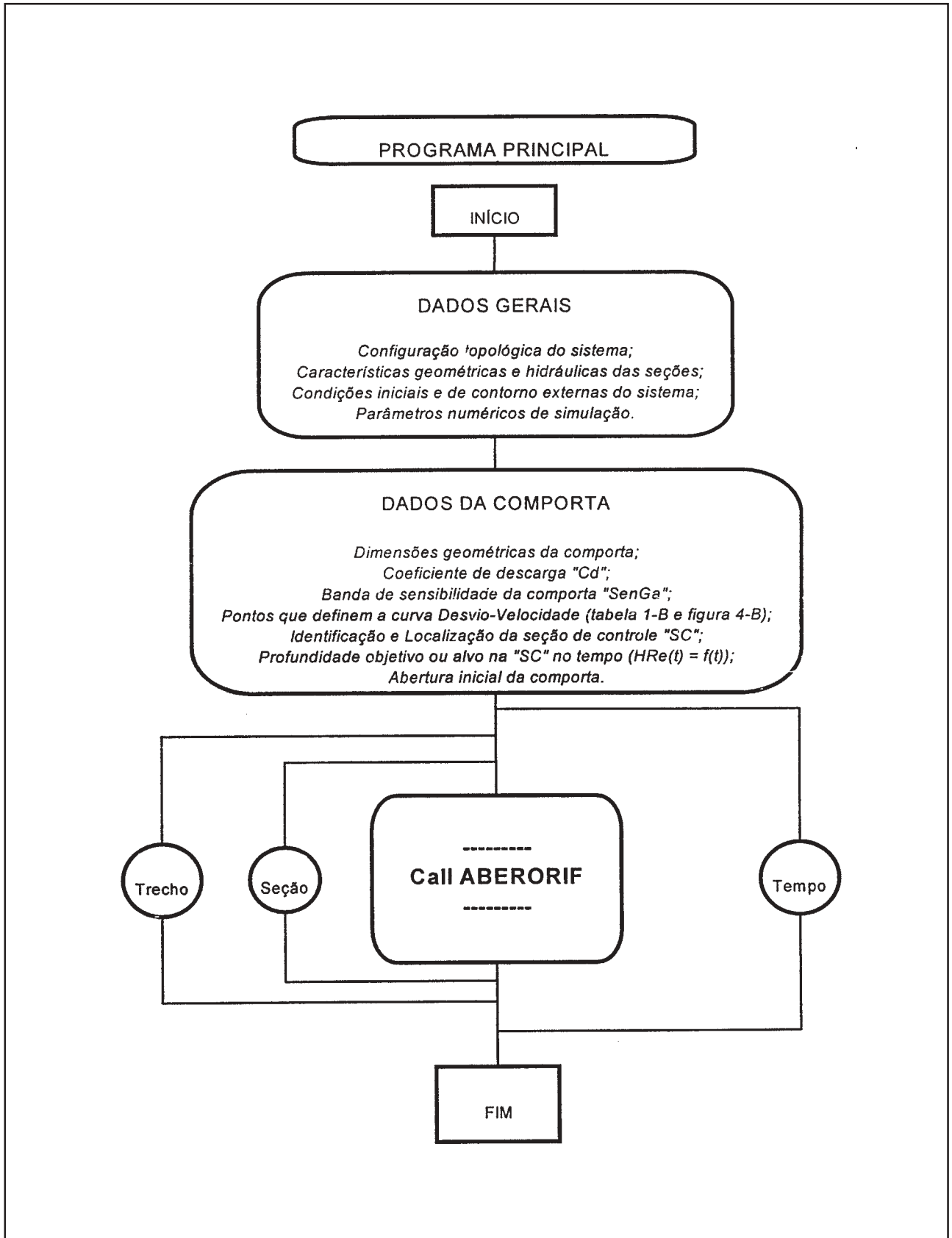
Figura 6. Fluxograma do algoritmo da comporta telecomandada.
